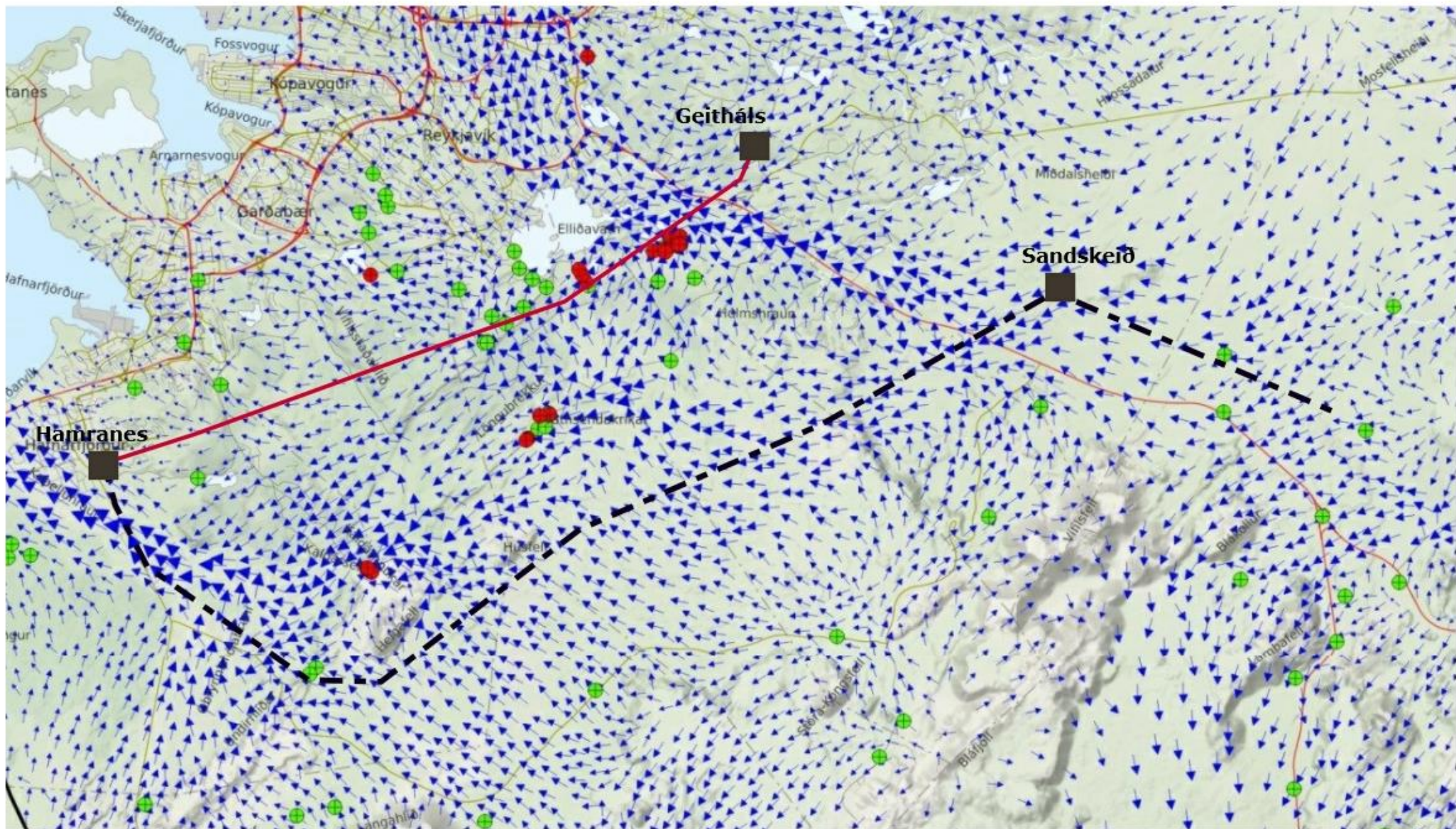
Mynd 1 Grunnvatnsstraumar skv. líkani Verkfræðistofunnar Vatnaskila. Örvarnar sýna rennsli grunnvatns, rauðir punktar brunnholur, svarta brotna línan sýnir legu Sandskeiðslínu 1 og rauða línan legu Hamraneslína að mestu norðan við grunnvatnsstraumana.
